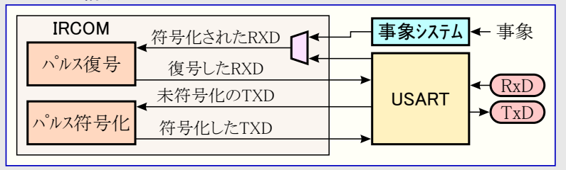
図25-13. 構成図
