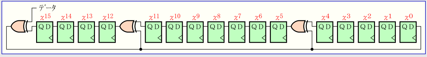
図28-2. CRC-16実装説明
