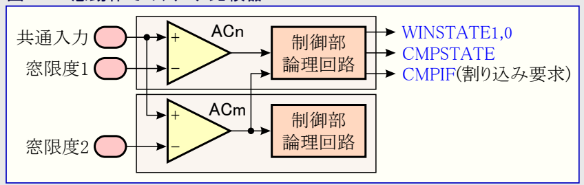
図30-2. 窓動作でのアナログ比較器
