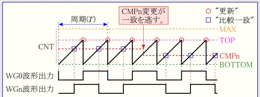
図22-10. 上昇計数時の変位
