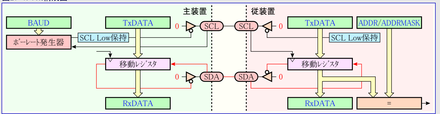
図27-1. TWI構成図
