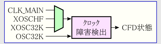
図12-3. クロック障害検出(CFD)構成図
