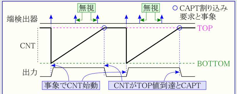
図23-9. 単発動作
