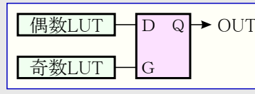
図29-9. Dラッチ
