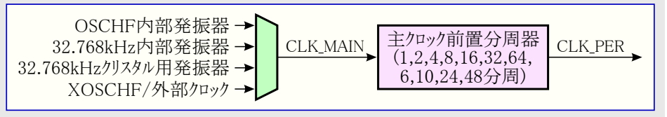
図12-2. 主クロックと前置分周器
