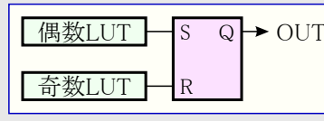
図29-10. RSラッチ
