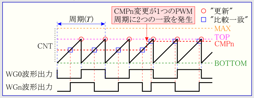
図22-11. 波形出力反転
