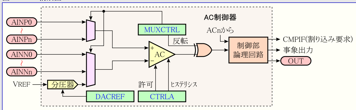
図30-1. AC構成図
